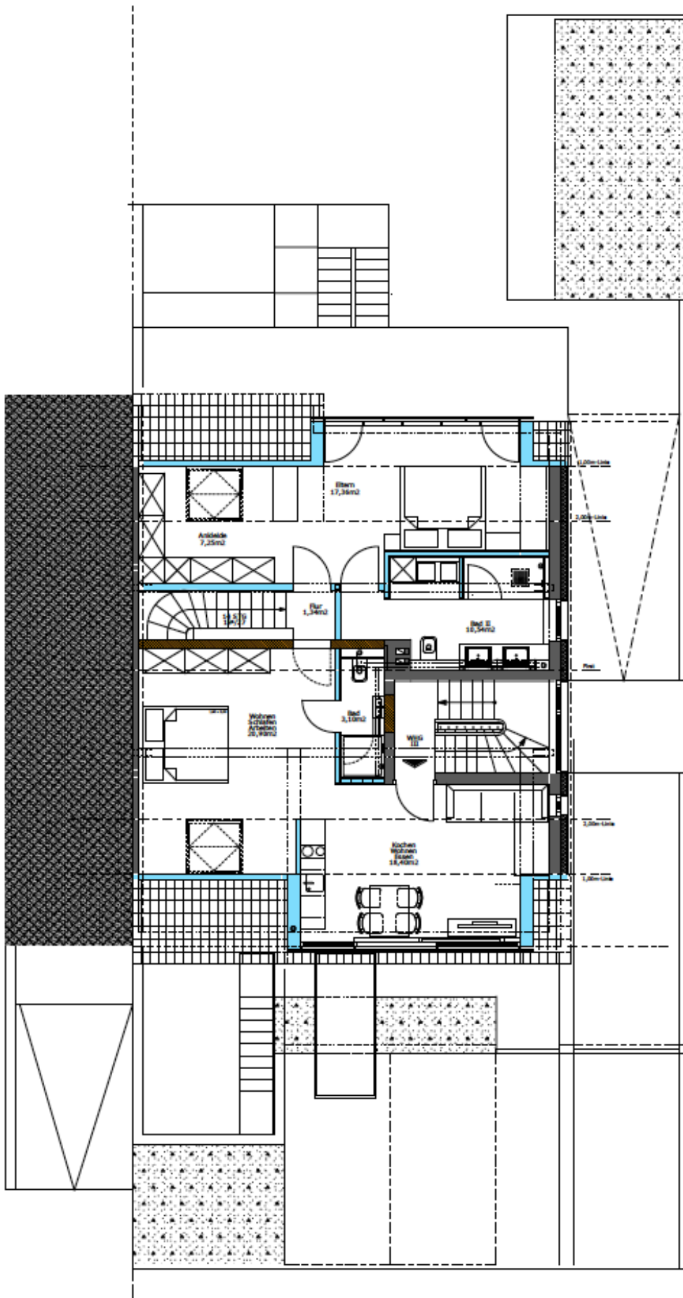
Grundriss DG
