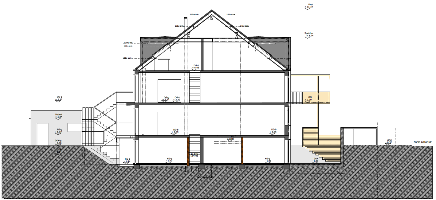
Gebüdeschnitt
