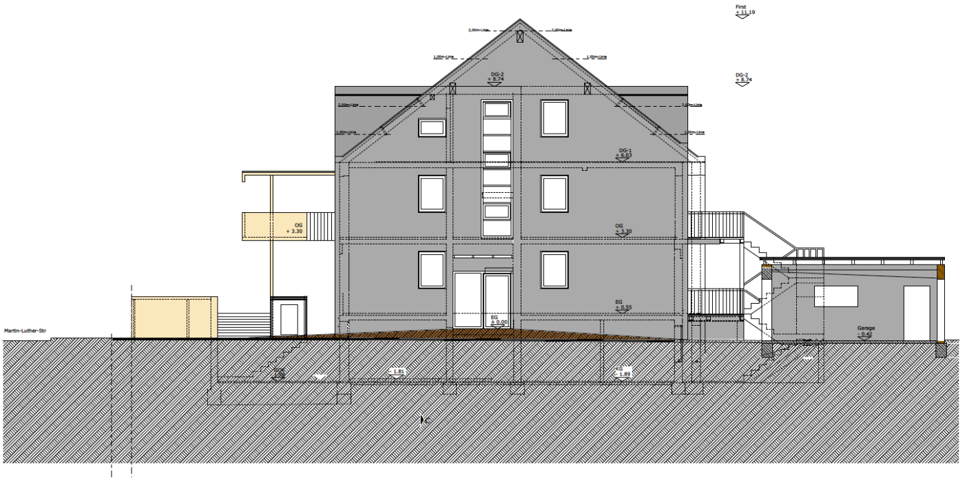
Ansicht Osten | Eingangsseite
